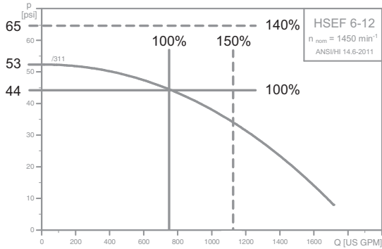
Рис. 15 Зависимость давления от подачи
