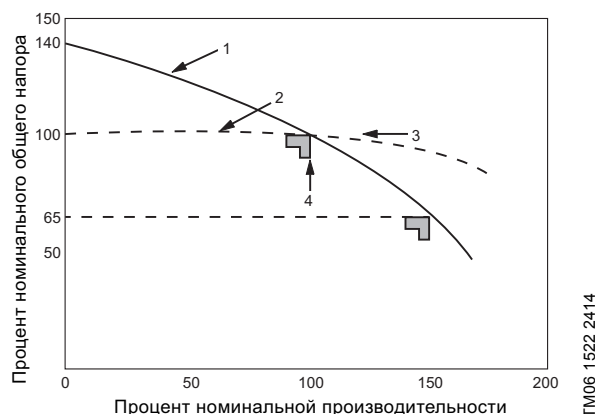
Рис. 14 Зависимость давления от подачи
