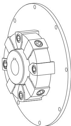
Рис. 17 Эластичная муфта
