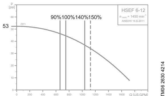
Рис. 18 Стандартный диапазон подачи
