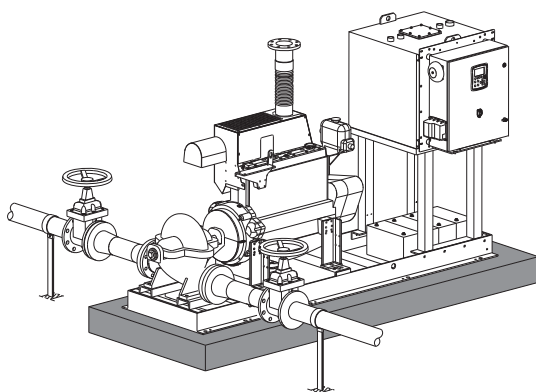
Рис. 4 Пример монтажа
