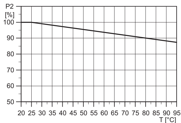
Рис. 20 Соотношение мощности двигателя (P2) и температуры окружающего воздуха
