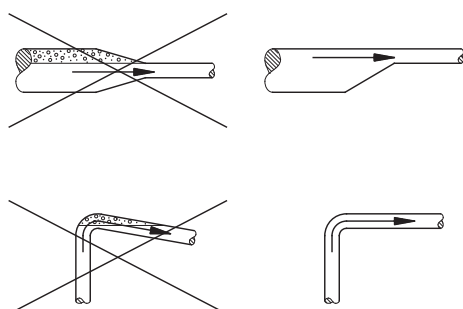
Рис. 22 Установка трубопроводов
