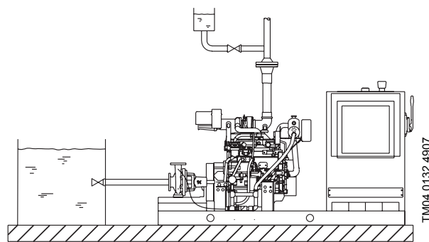
Рис. 18 Схематическое изображение открытой системы с насосом NKF
