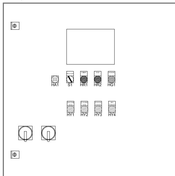
Рис. 8 Прибор управления пожарными насосами Control MX
